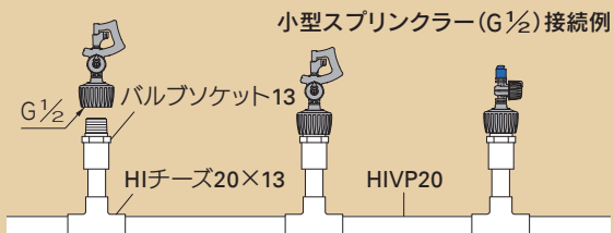
小型スプリンクラー(G \frac{1}{2} )接続例
