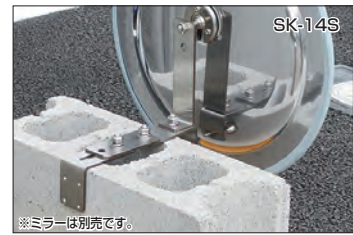
〈取付け図〉〈構造図〉
