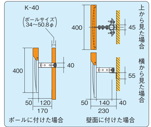
〈取付け図〉〈構造図〉
