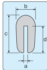
〈構造図〉 H-03
