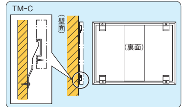
〈取付け図〉〈構造図〉
