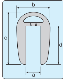
〈構造図〉 H-08~22
