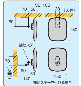
〈取付け図〉
