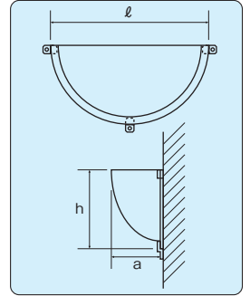
〈取付け図〉
