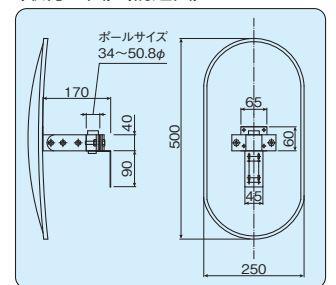
〈取付け図〉〈構造図〉
