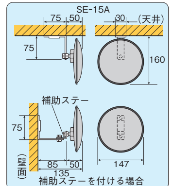
〈取付け図〉〈構造図〉
