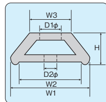
〈構造図〉
