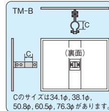
〈取付け図〉〈構造図〉
