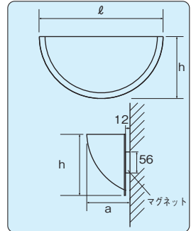
〈取付け図〉
