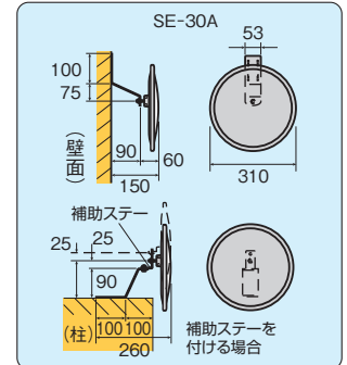
〈取付け図〉
