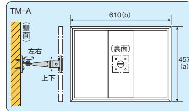
〈取付け図〉〈構造図〉
