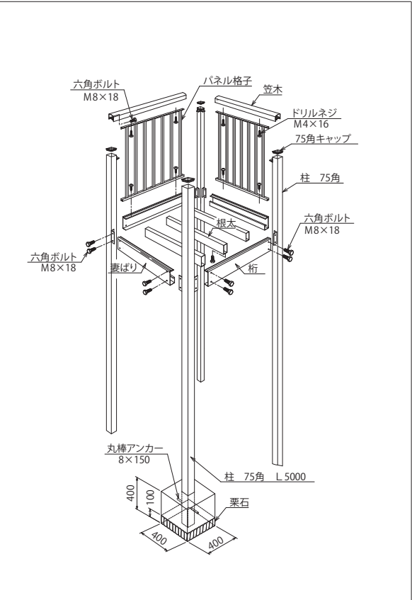
Dタイプ踊場
