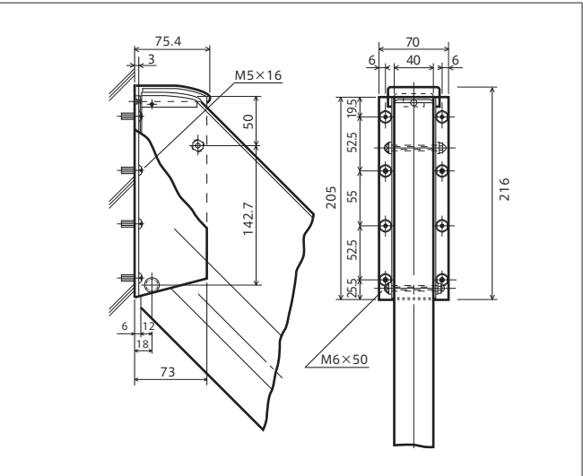
サイドフレーム 上部取付詳細
