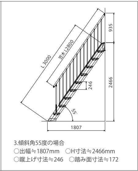
基本図 斜角 55°
