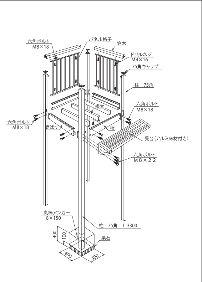
Bタイプ踊場
