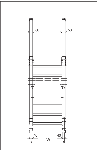
正面図
