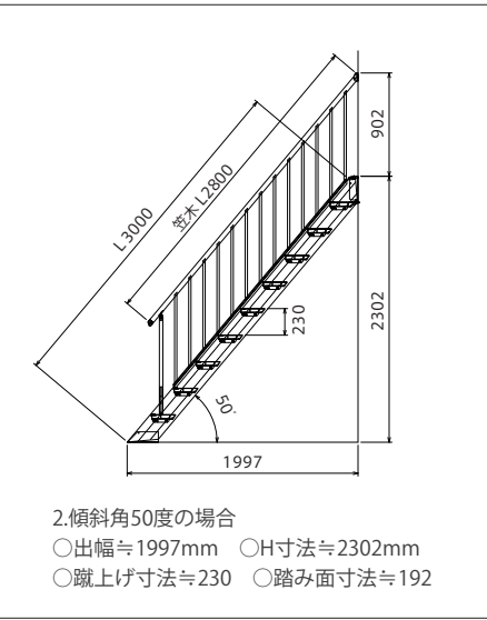
基本図 斜角 50°
