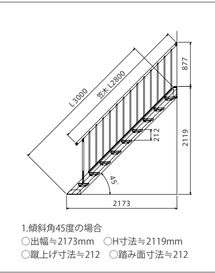
基本図 斜角 45°
