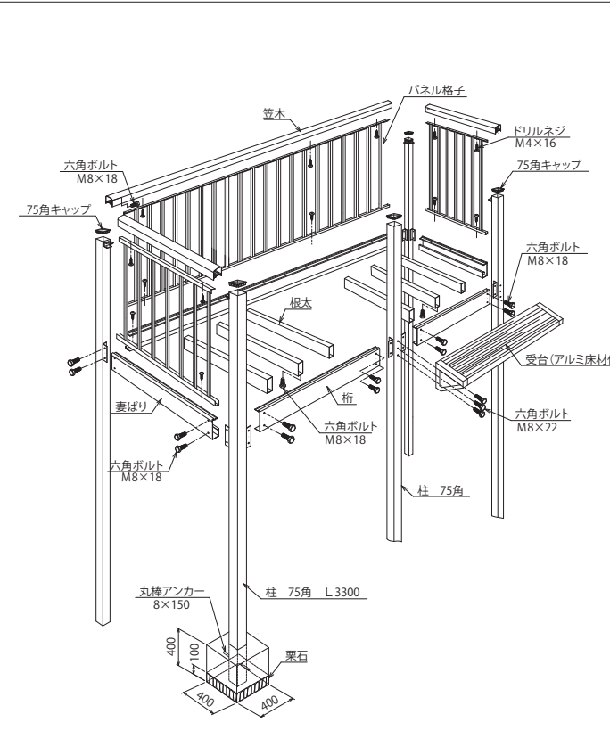
Cタイプ踊場
