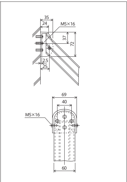
手摺取付部詳細
