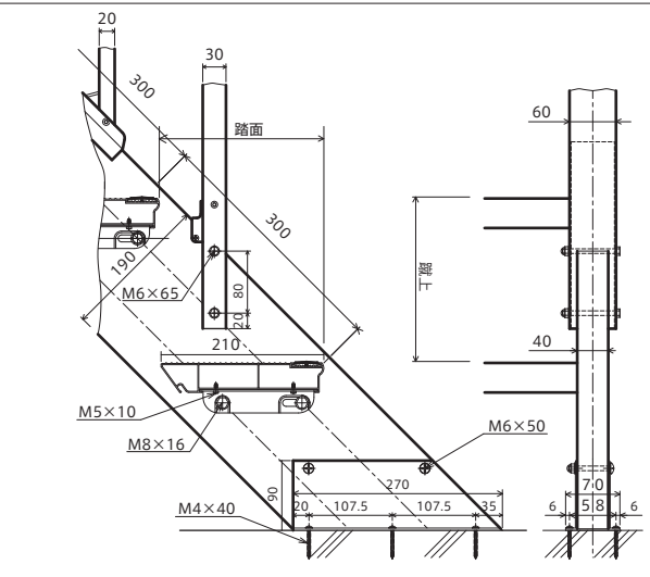
サイドフレーム 下部取付詳細
