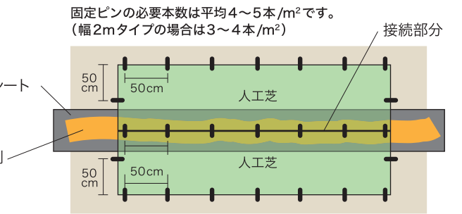
図② 人工芝をピンで固定する
